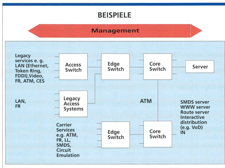
Bild 7. Lösungsbeispiel eines ATM-Netzes.
