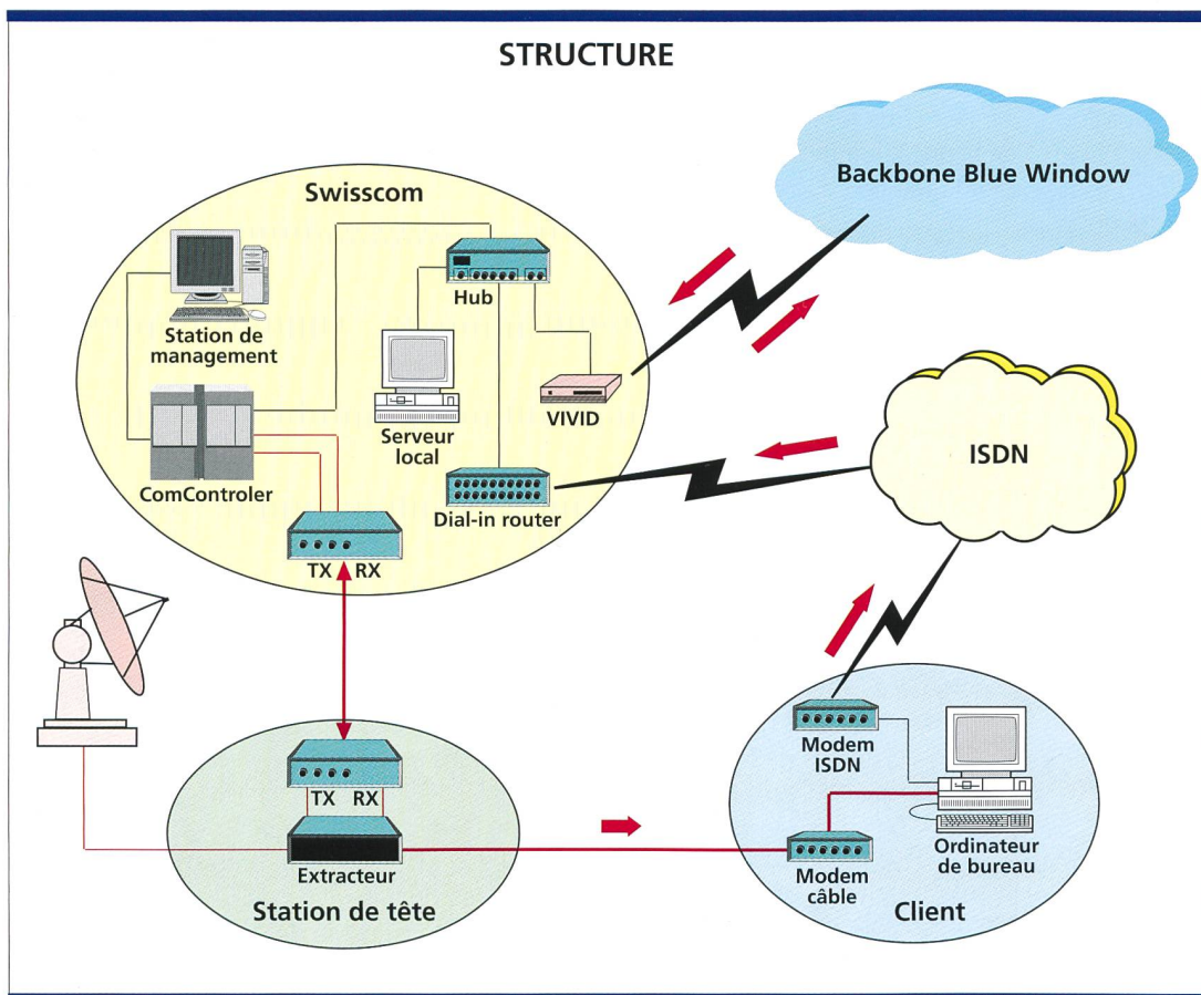
Figure 3. Structure du réseau avec la voie de retour téléphonique.
