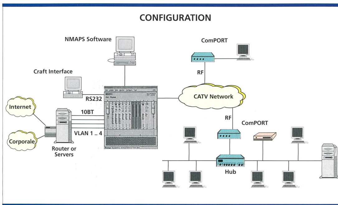
Figure 9. Configuration détaillée retenue pour les essais.
