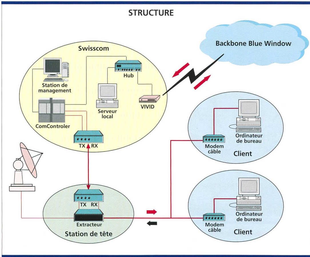
Figure 2. Structure du réseau avec voie de retour CATV.
