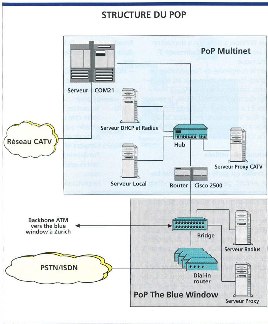
Figure 4. Structure générale du PoP Multinet connecté sur le PoP Blue Window.
