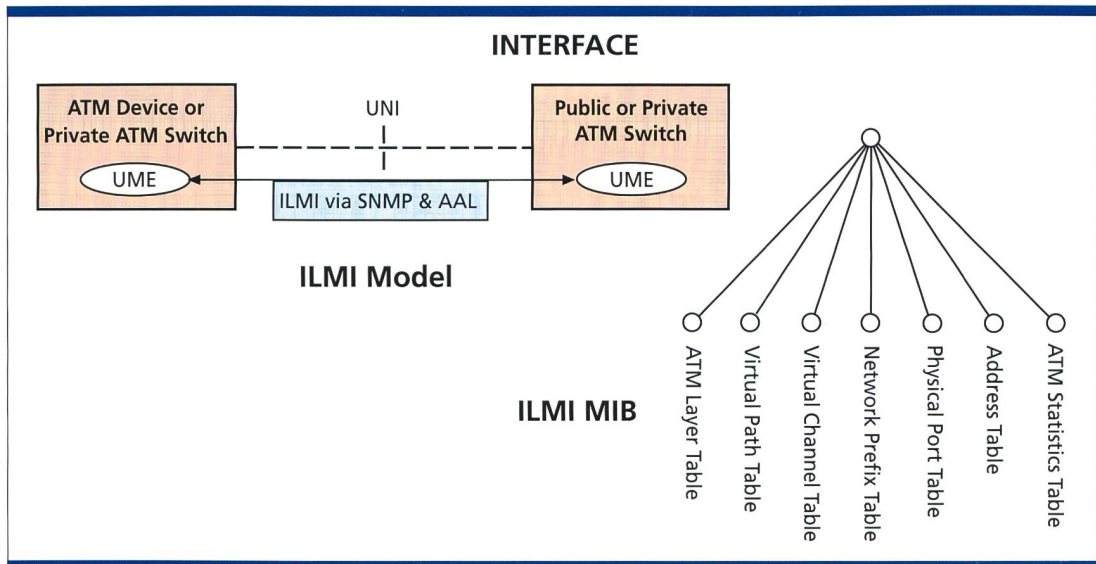
Bild 6. ILMI (Interim Local Management Interface) des ATM-Forums.
