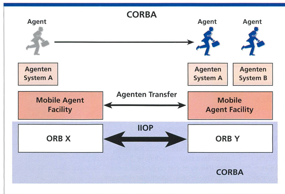
Bild 16. CORBA als Basis Mobiler Agenten.
