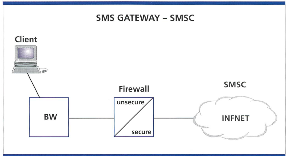
Bild 2. Schema der Verbindung vom SMS Gateway via Firewall zum SMSC.
