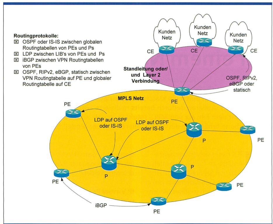
Bild 2. Zusammenspiel der verschiedenen Routingprotokolle in einem MPLS/VPN-Netz.
