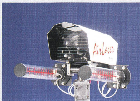
AirLaser IP100 mit integriertem Backup-System und den zwei Antennen im 2,4-GHz-Bereich.
