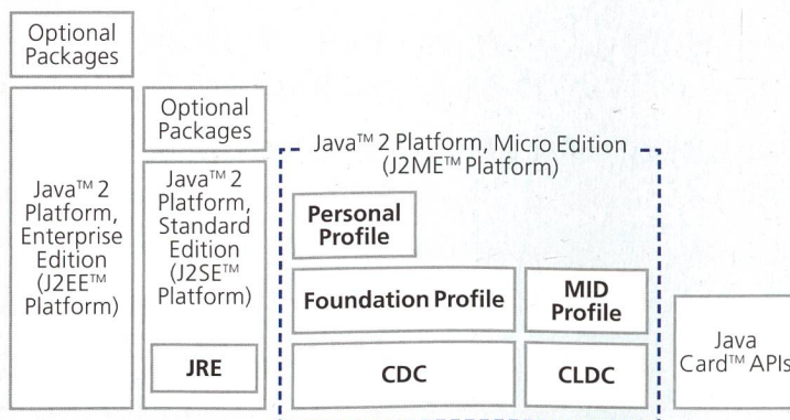
Bild 1. Übersicht: Java-Plattform.
