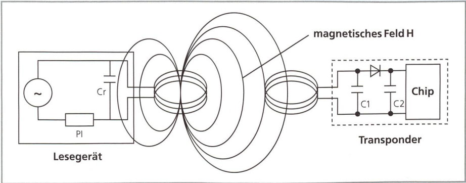
Bild 4. Wenn eine Spule aus einem leitfähigen Material in einem Wechselfeld eingebracht wird, entsteht ein Stromfluss in der Spule.
