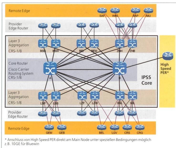
Bild 6. Layer-3-Topologie, basierend auf einem CRS-1 Router von Cisco Systems.
