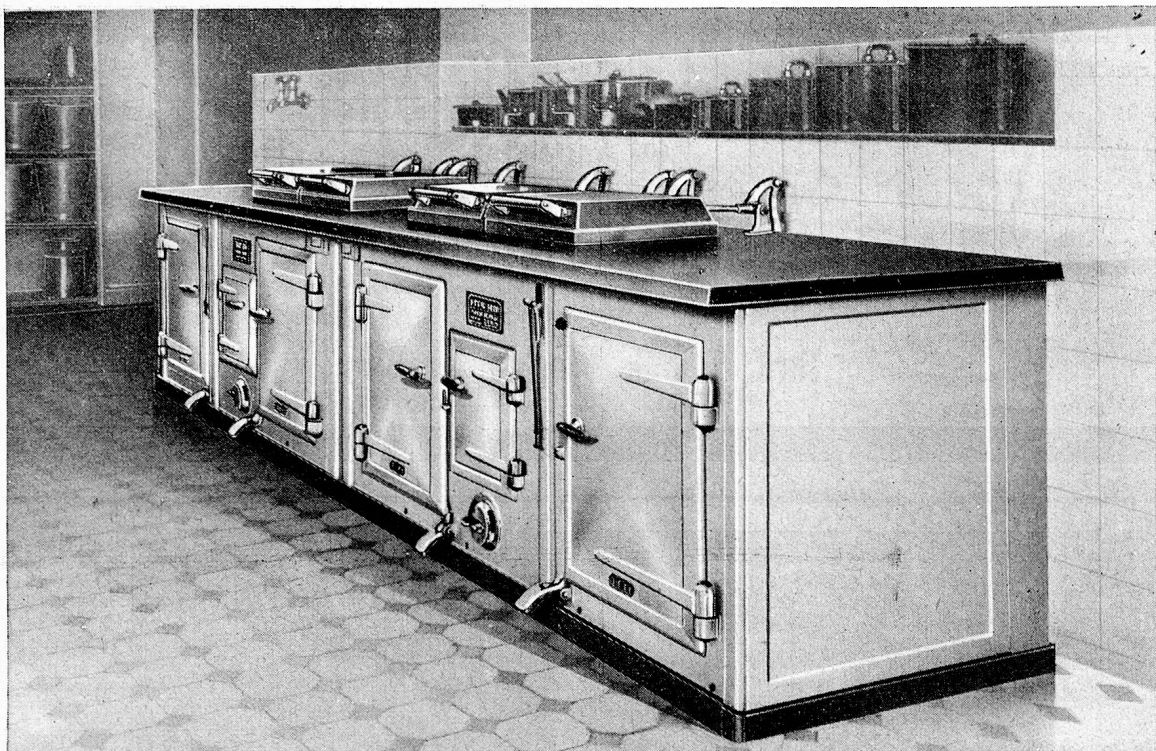
ESSE-Großküche in der kant. Heil- und Pflegeanstalt St. Pirminsberg, Pfäfers. Major-Doppelherd von 4 m Länge mit 4 Brat-, Back- und Kochschränken, für ca. 400 Personen.
