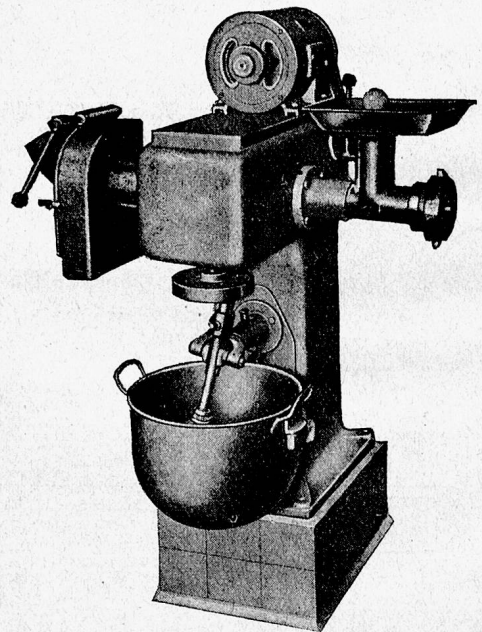
KÜCHENMASCHINE
