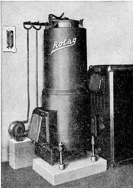
„ROTAG“-Vorbaubrenner
