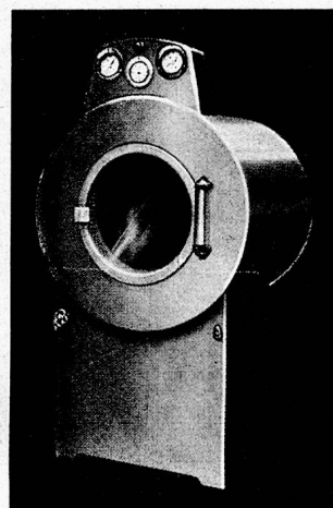
Wäsche-Tumbler (Wäschetrockner) 45 kg Trockenwäsche pro Stunde
