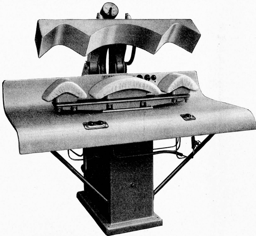
Modell PWE-67, Kragen- und Manchettenpresse
