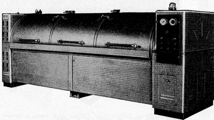
Aus unserem Erweiterungsprogramm eine der neuen Klarstrommaschinen (Syst. Sulzmann) 1. und 2. Stufe in Pullmannausführung, Gesamtfassung 150 kg
