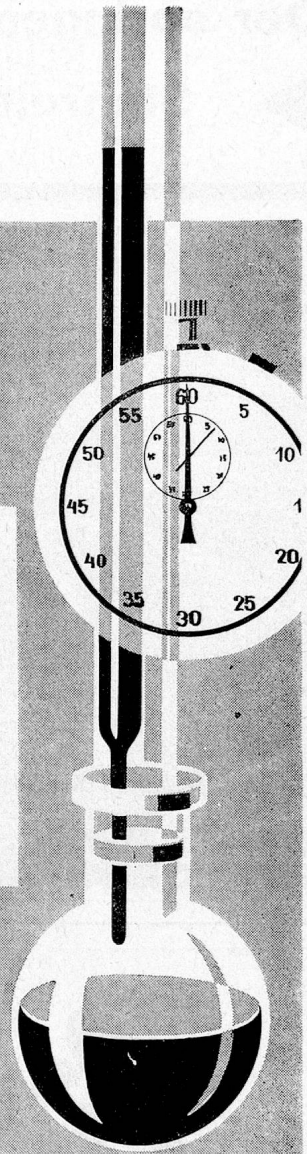
Prüfung des chemischen Abbaus der Zellulose
