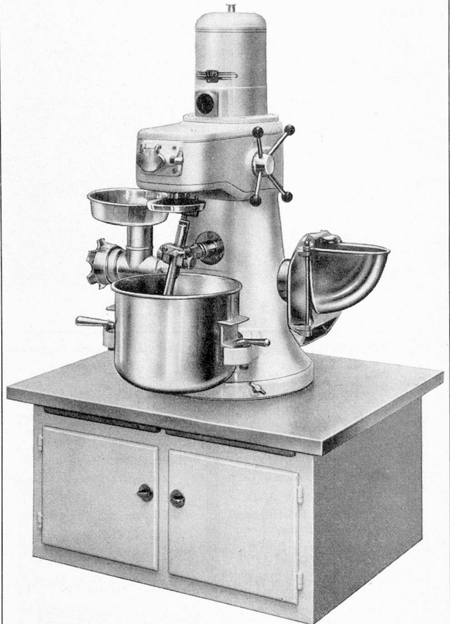
Combirex-Maschine, drehbar
