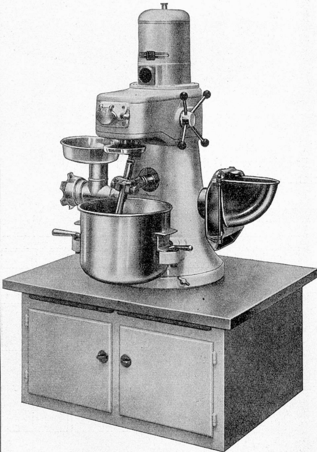
Combirex-Maschine, drehbar
