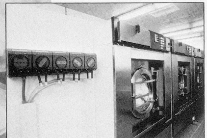
Eine moderne Grosswaschanlage: 600 Liter «Clarax Profi»-Container, Claramatic- Dosierpumpen und Grosswaschmaschine.
