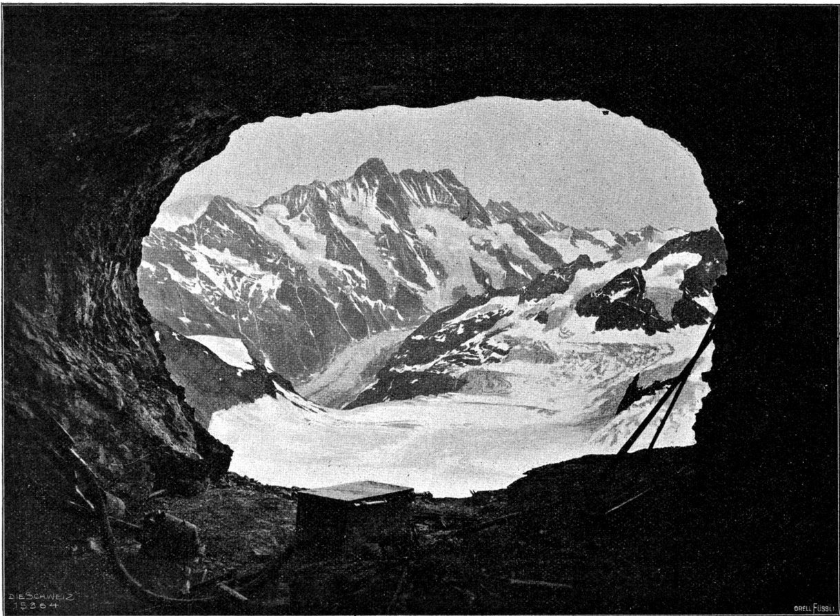
Ausblick von Station Eismeer auf die Schreckhörner etc. (Phot. Gebr. Wehrli, Mischberg).
