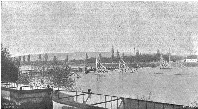
Zentraleurop. Binnenschifffahrt. Die Hünzler Schiffsbrücke. Das über die Gerüste gespannte Drahtseil dient zum Ausfahren einzelner Brückenteile zur Ermöglichung der Durchfahrt.
