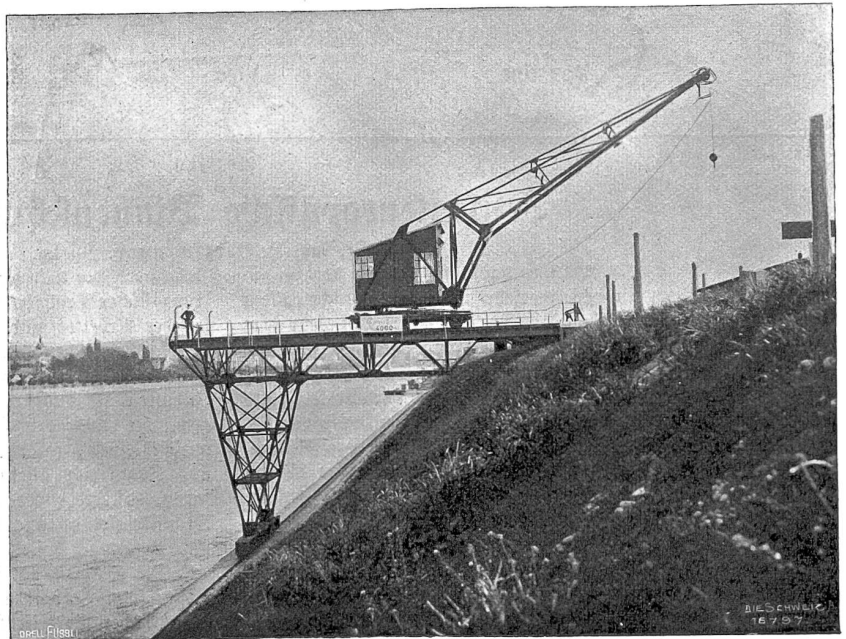
Zentraleurop. Binnenschifffahrt. Verschiebbarer Kran zum Ein- bzw. Ausladen der Rheinschiffe auf dem Hafenhof der S. B. D. zu Basel.
