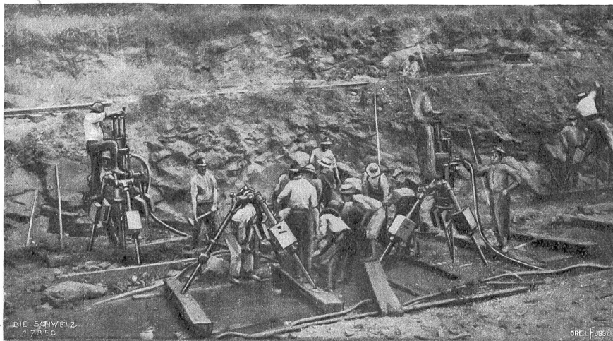
Vom Panama-Kanal Abb. 4. Jagerfoll-Druckluftbohrmaschinen.
