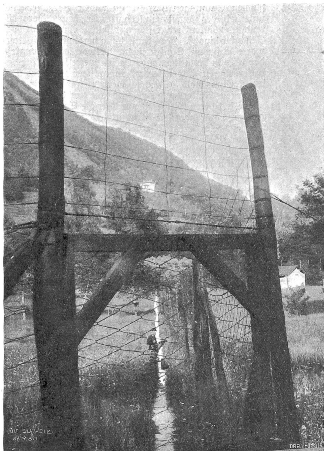
Drachtgeflecht mit Stöcke und Durchlaßtür an der schweizerisch-italienischen Grenze.
