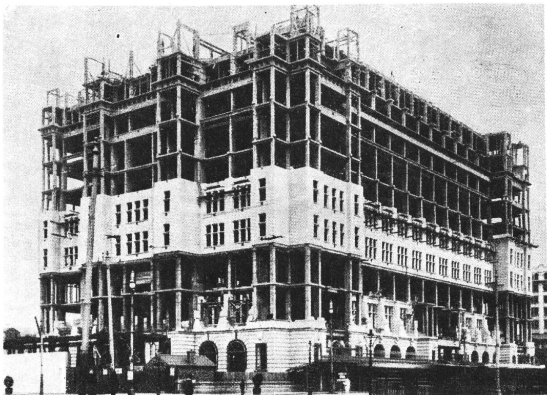
Fig. 12. — «Royal Liver Building», Londres, 1909. L. G. Monchel & Partners, ingénieurs; W. A. Thomas, architecte. Image de l'ossature en voie d'habillement. Reconduction de la maçonnerie «traditionnelle» et de ses règles de composition.
