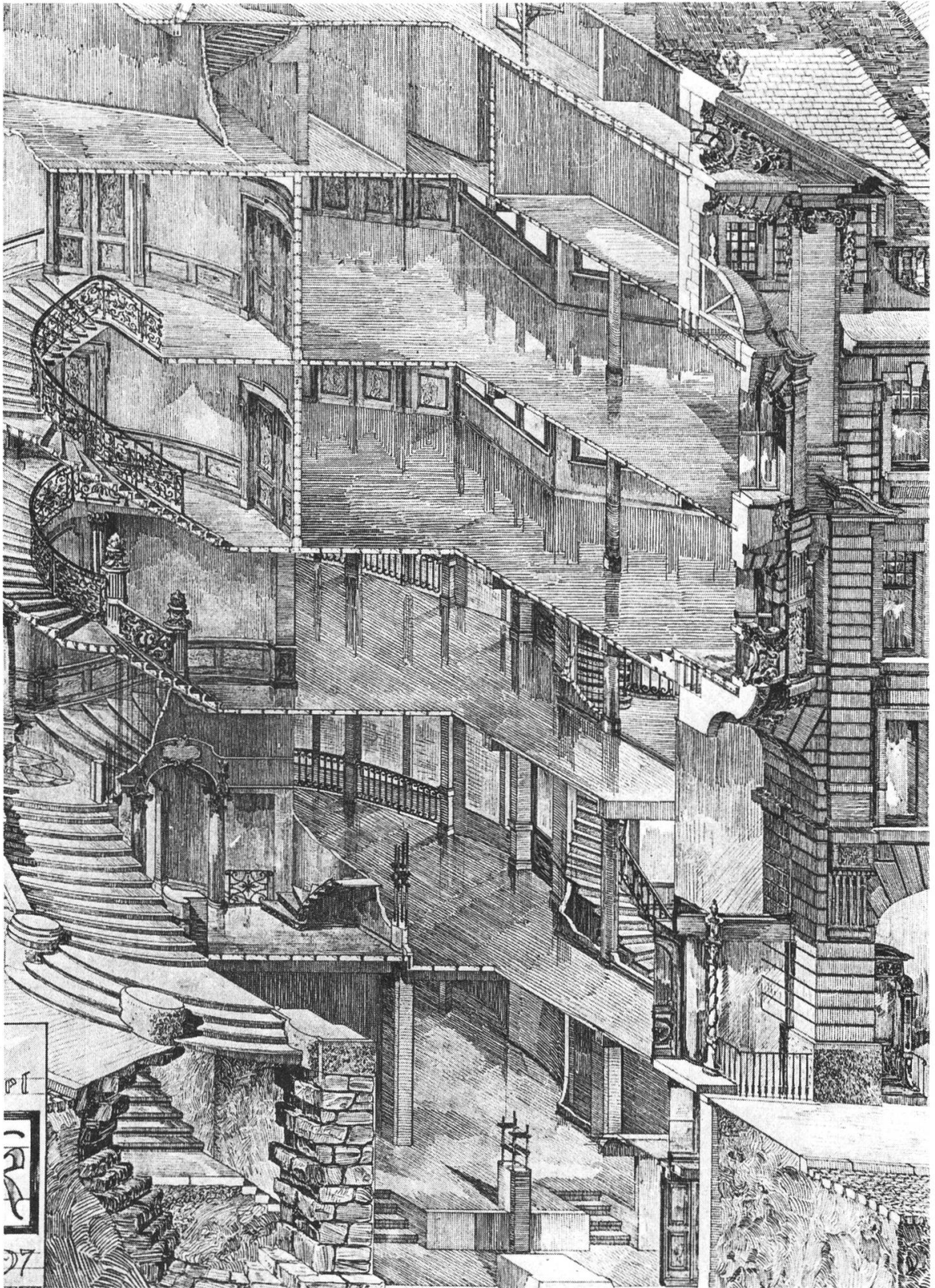
Fig. 15. — Coupe perspective de l'immeuble administratif «Zum Sodeck» à Bâle, dessin de l'architecte-entrepreneur-concessionnaire Rudolf Linder, œuvre des années 1896 et 1897.
