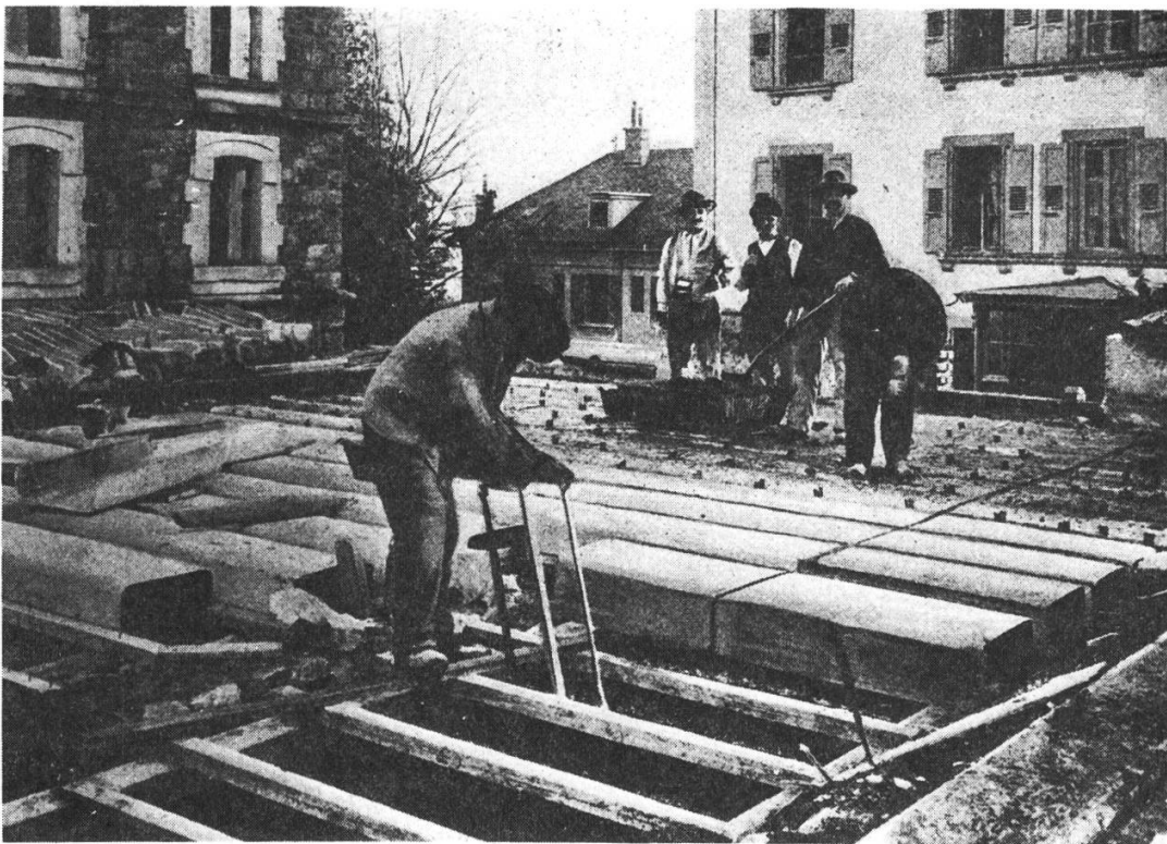
Fig. 25. — Lausanne, 1904. Construction d'un plancher Hennebique. Récupération des coffrages métalliques, selon une mise au point de l'ingénieur Samuel de Mollins et de la concessionnaire A. Ferrari.
