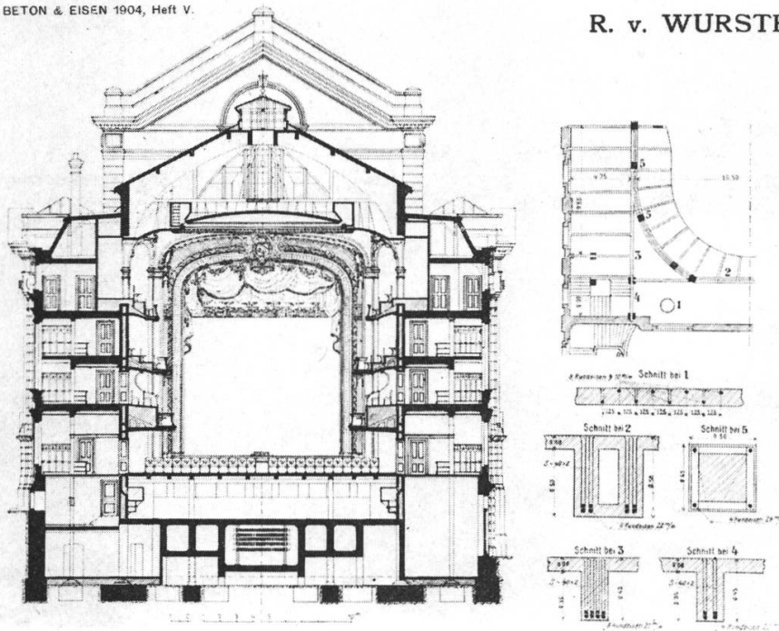
Fig. 16. — Théâtre de la Ville de Berne, 1897-1903. Samuel de Mollins, ingénieur; R. von Wurstenberger, architecte; Anselmier et Gautschi, entrepreneurs-concessionnaires. Bel immeuble incombustible.
