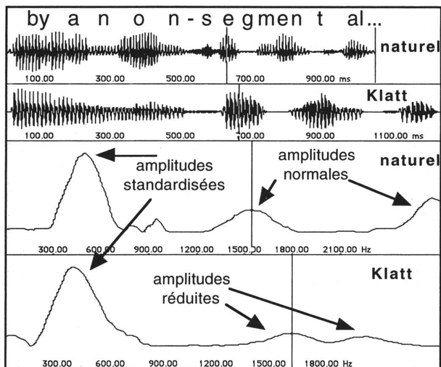
Figure 5. Comparaison de spectres pris sur la voyelle / \epsilon / de non-segmental synthesis system . Haut: locuteur humain. Bas: synthèse par formants, méthode de Klatt adaptée à l'Université de York, UK. Les pics des formants 2 et 3 de la synthèse sont fortement réduits, en comparaison avec les pics du spectre naturel. La représentation du Formant 1 a été standardisée à la même hauteur par le logiciel d'affichage graphique.
