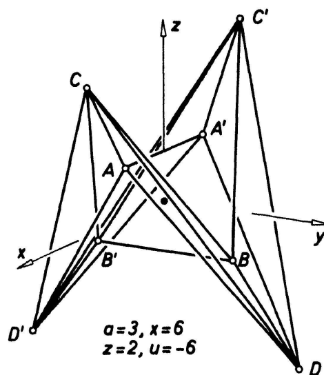
Figur 3. Überschlagenes Wackeldodekaeder I. Art.
