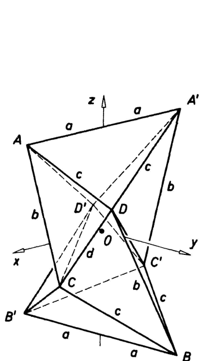
Figur 1. Doppelt-symmetrisches Kipp-Dodekaeder.
