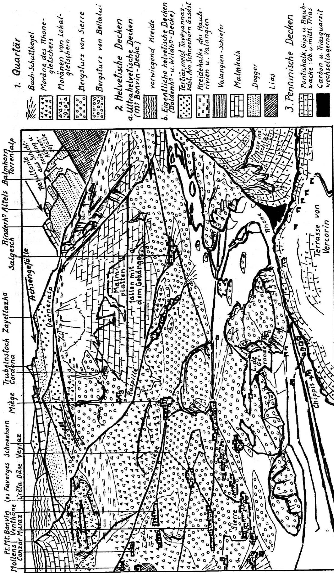
FIG. 2. — Traduction des légendes. — 1° Quaternaire : cônes d'alluvions de torrents ; moraines du glacier du Rhône ; moraines de glaciers locaux ; éboulement de Sierré ; éboulement de Bellalut. 2° Nappes helvétiques : a) nappes ultrahelvétiques (nappe du Mont Bonvin) ; crétacé dominant ; b) nappes helvétiques
