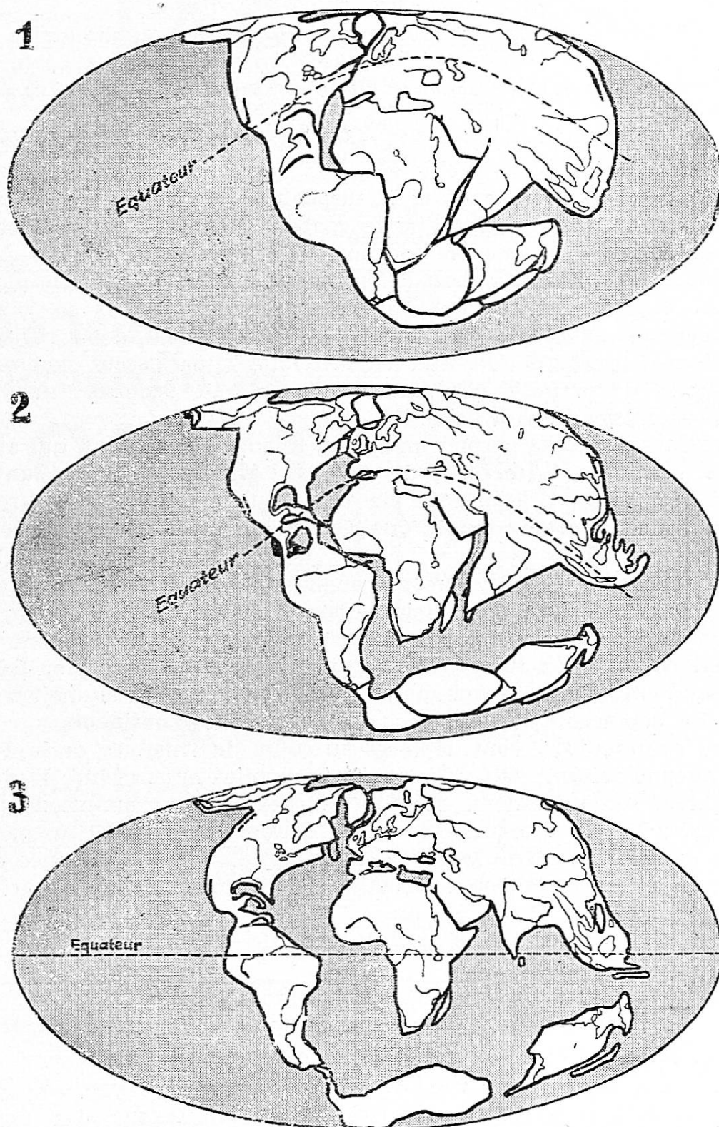
La situation des continents : 1. A la période carbonifère, ère primaire ; 2. Au début de l'ère tertiaire ; 3. Au début de l'ère quaternaire. D'après Wegener. (Document Gilde du Livre.)
