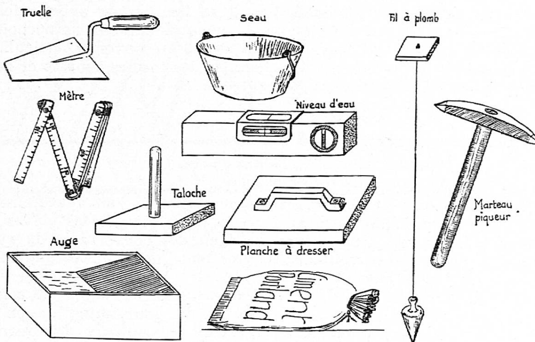
Les outils du maçon-manoœuvre.
