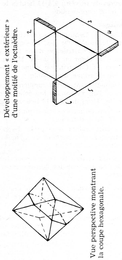
Fig. 4. L'octaèdre.
