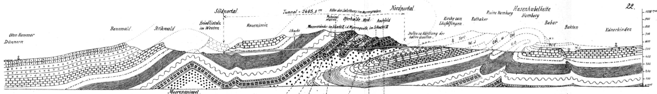
Profil von Otten-Hammer über den Hauenstein-Tunnel, den Hornbühl bis Bukten aufgenommen von F. Mühlberg 1889
