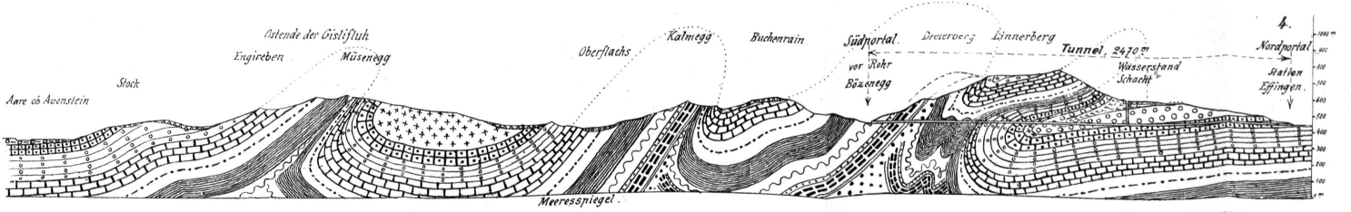
Profil von Auenstein nach Bözeneq und durch den Bözberg-Tunnel von F. Mühlberg.
