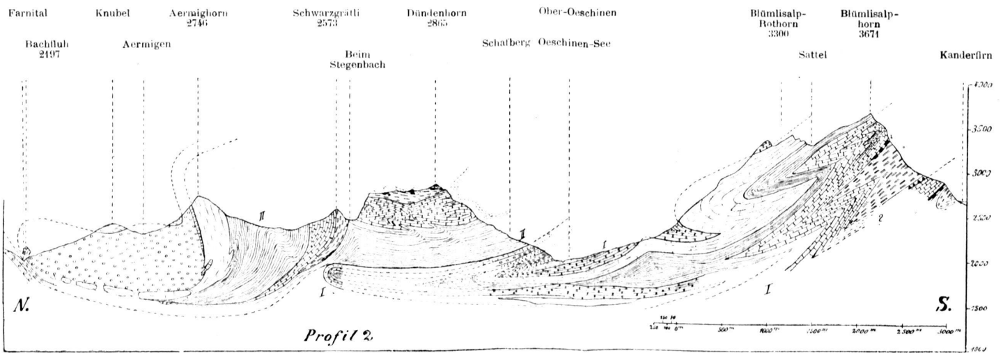
Profile durch die westlichen Kientaleralpen. I. Innere Kalkalpen (Basis). II. Mittlere Kalkalpen (Decke).
