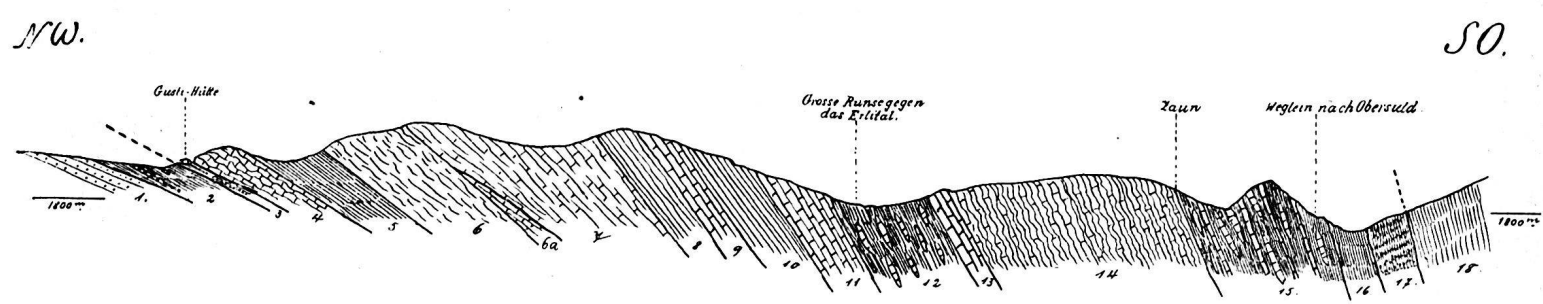
FIG. 10. — Schichtfolge der Klippengesteine auf dem Rengg-Alp-Grat.
