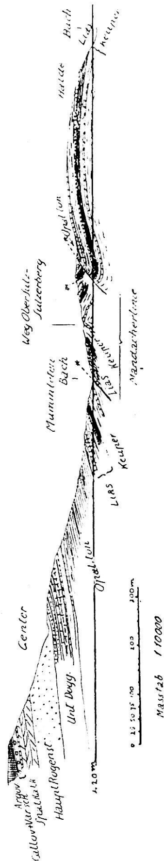
Fig. 9. — Dislokationen an der Mandacherlinie bei Ober-Sulz.
