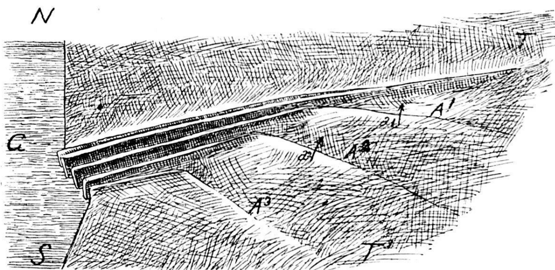
FIG. 6. — Modellzeichnung zur Veranschaulichung der Entstehung der südlichen Antiklinalen ( A' bis A^3 ) am östlichen Juraende, wo die auf einer festen Unterlage G nordwärts geschobene Tafel T^1 nach E in die in Ruhe verharrende Tafel T übergeht.
