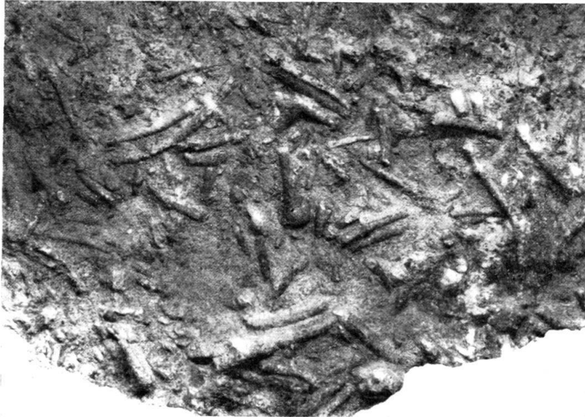
Dentalien vom Gurten.
