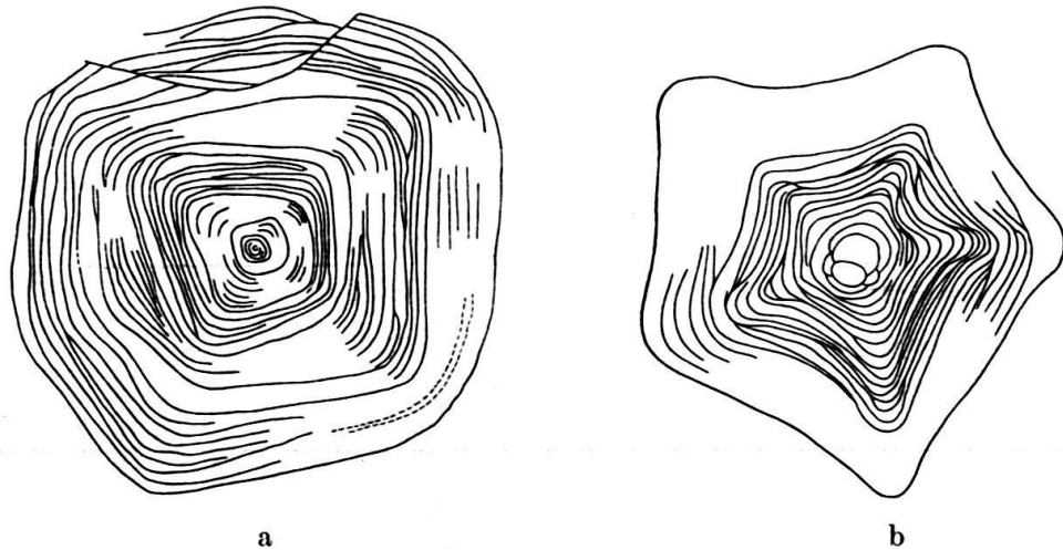
Fig. 1. Vergleich der Entwicklungsstadien des Umrisses der A- und der B-Generation von Asterocyclusen.
