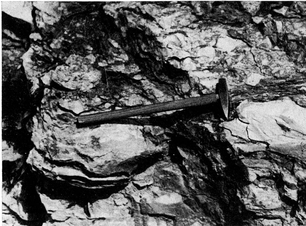
Fig. 12. Ausbildung der Wangbreccie, Rothornweg, S Wilerhorn, bei 1650 m.
