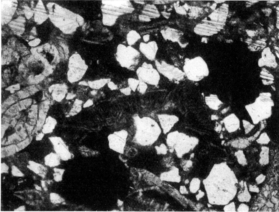
Fig. 3. Fabiania SILVESTRI. 25 \times vergr. (Zentrum des Bildes), Kalkiger Sandstein. Bach 220 m nordwestlich Hohmädli, Q. 1305.
