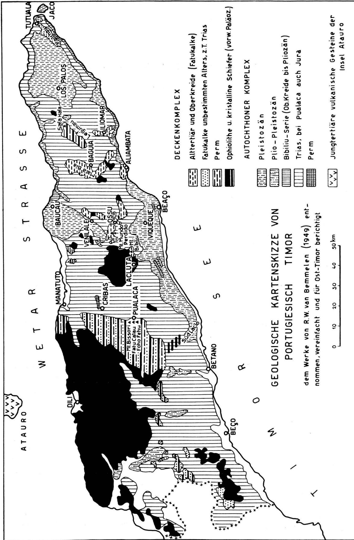
Fig. 1 Berichtigung: Die beiden Antiklinalen 20 km WSW von Viqueque sind 10 km nach ENE verschoben zu denken.
