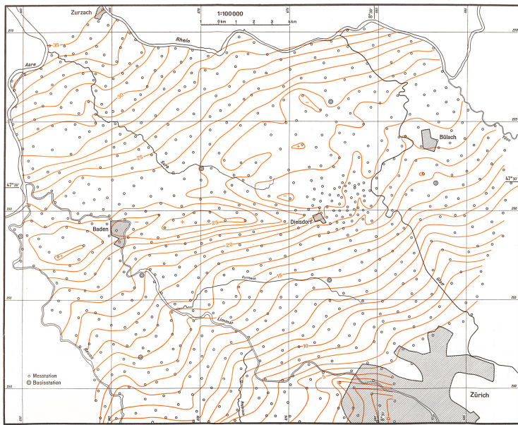
«BOGUERKARTE I» Kurven gleicher Werte von u_1 in mg/l.
