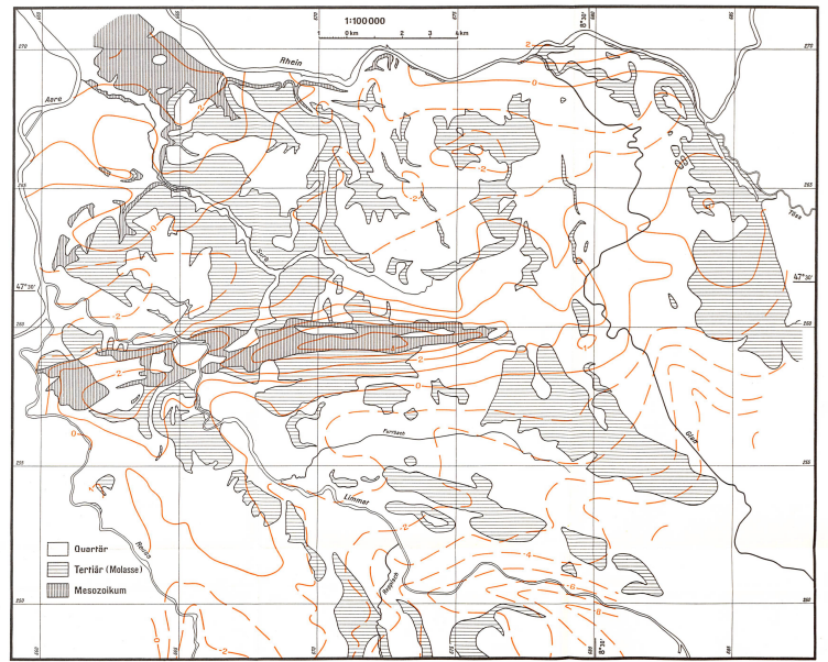
«BOGUERKARTE II» Kurven gleicher Werte von u_2 in mg/l.
