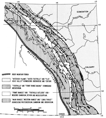
TEKTONISCHE ÜBERSICHTSKARTE DER ROCKY MOUNTAINS
