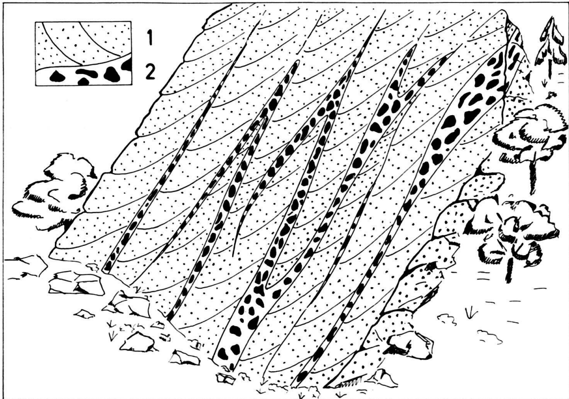
Fig. 2. Exemple de stratification entrecroisée: Paroi au S de Dorénav. 1 = Grès, 2 = Poudingue de Vallorcine
