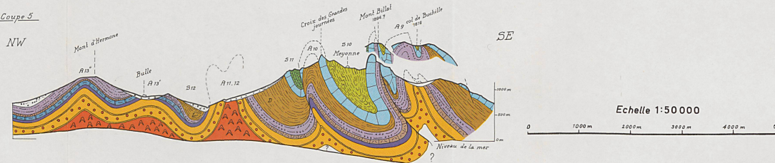
Coupe 5
