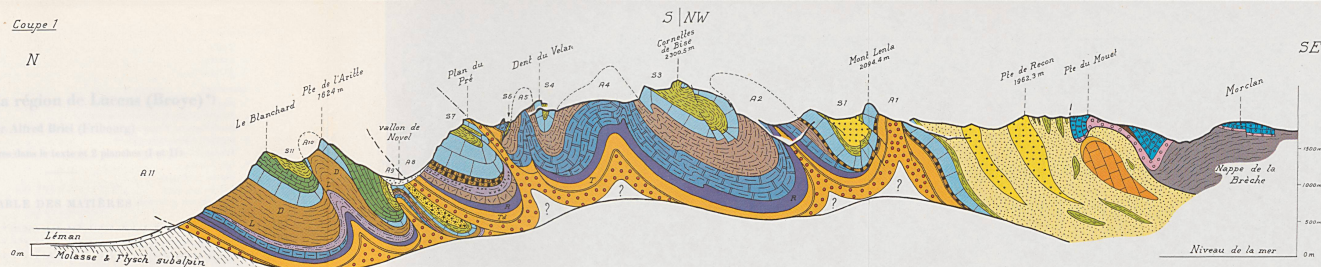
Coupe 1
