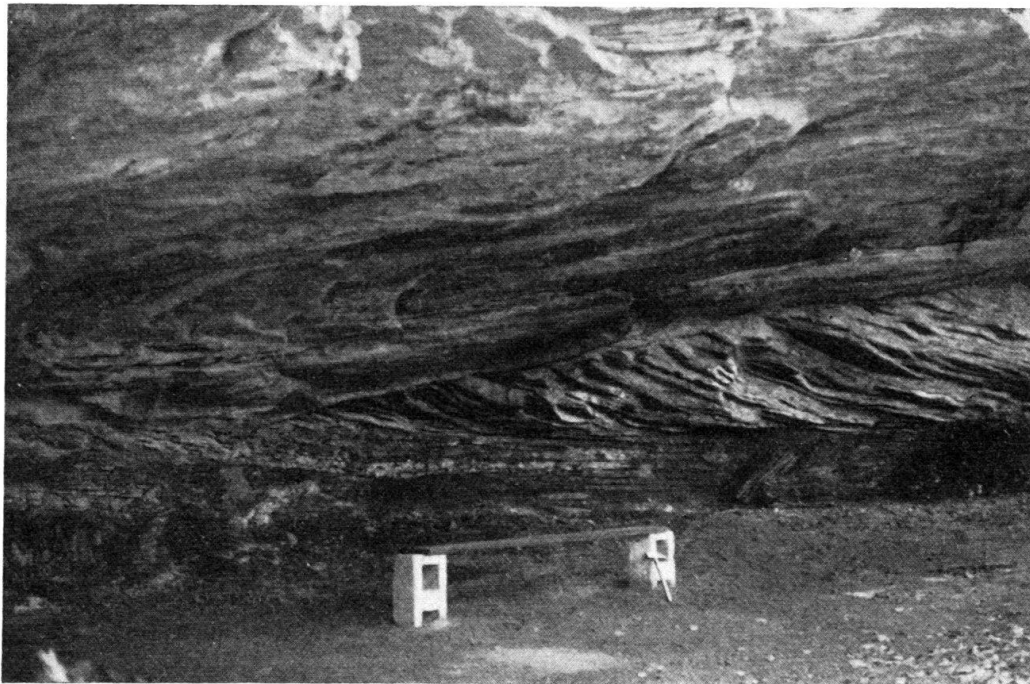
Fig. 12. Stratification entrecroisée. Molasse marine supérieure. Les Marchets, au SEE de Combrement le Grand.
