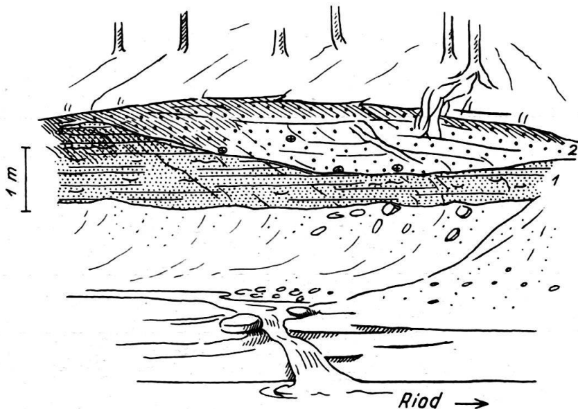
Fig. 11. Chenal d'érosion remblayé. Molasse marine supérieure. Rioid, au SE de Combremont le Grand.
