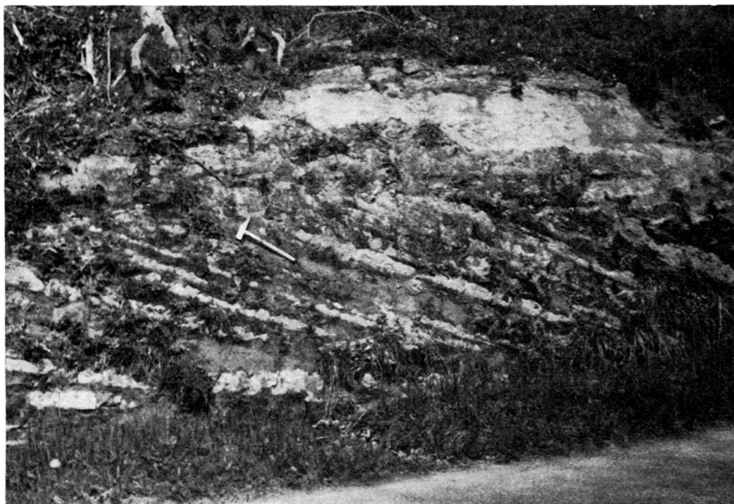
Fig. 21. Faciès des grès à stratification oblique. Lucens, route de Cremin.
