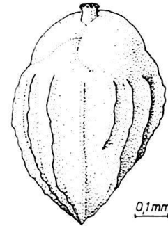
Fig. 23. Uvigerina eocaena GÜMBEL
