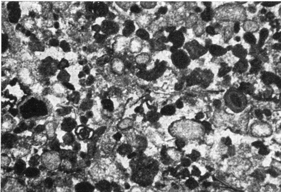
Fig. 5. Dolomie oolithique du type b). A remarquer: 1. une oolithe a conservé la structure concentrique; 2. la présence d'un Miliolidae . Grossissement: 30 ×
