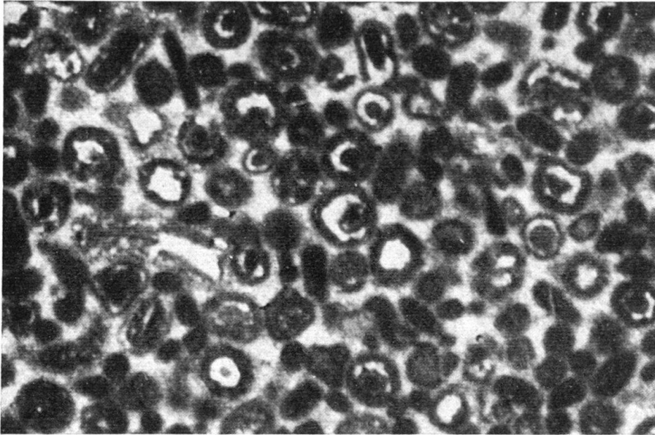
Fig. 4. Dolomie oolithique du type a). Grossissement: 30 ×
