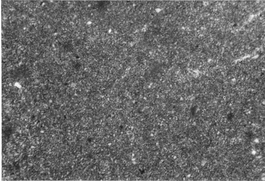
Fig. 3. Dolomie cryptocristalline. Grossissement: 72 ×
