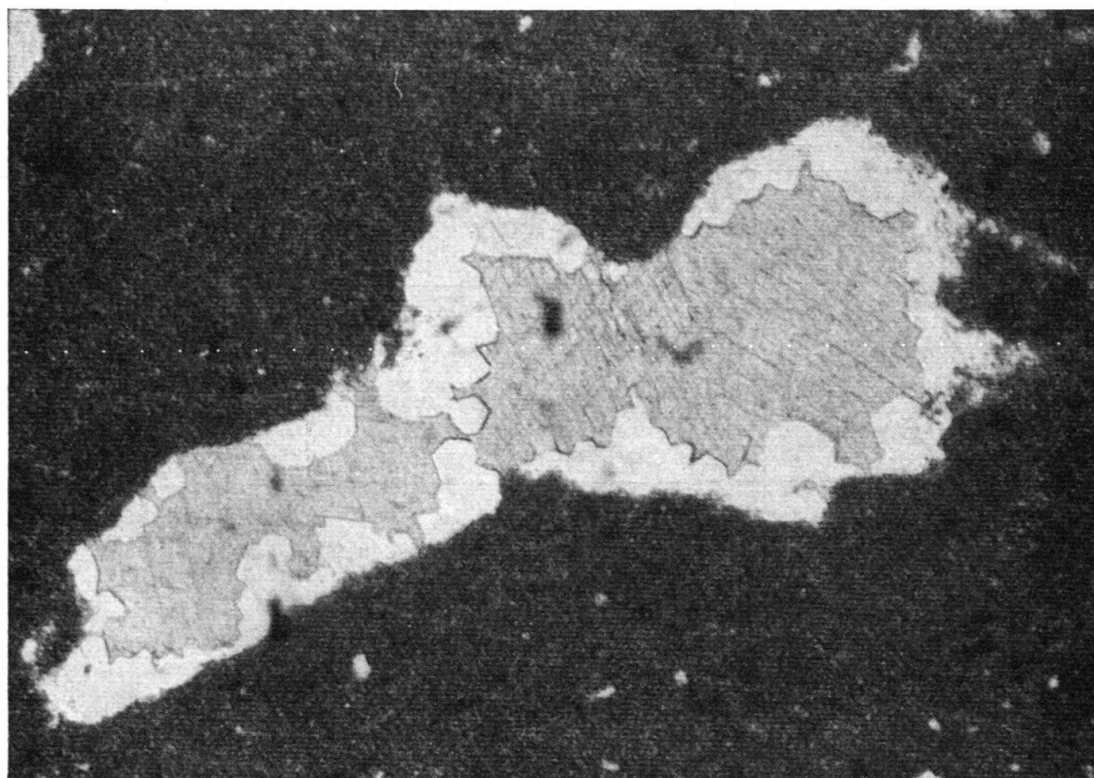
Fig. 7. Relique de calcite (au centre) fortement attaquée par la silicification (liséré blanc) et par la dolomitisation (masse sombre de dolomie cryptocristalline). Grossissement: 56 ×
