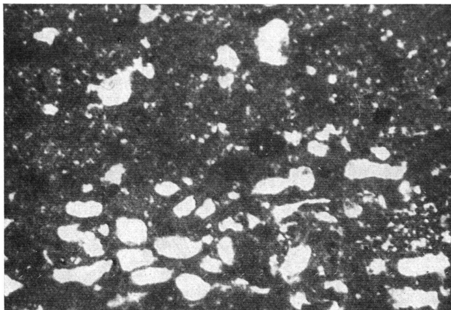
Fig. 6. Agrégats de quartz secondaire (taches blanches) dans une dolomie microgrenue à cryptocristalline. Grossissement: 30 ×
