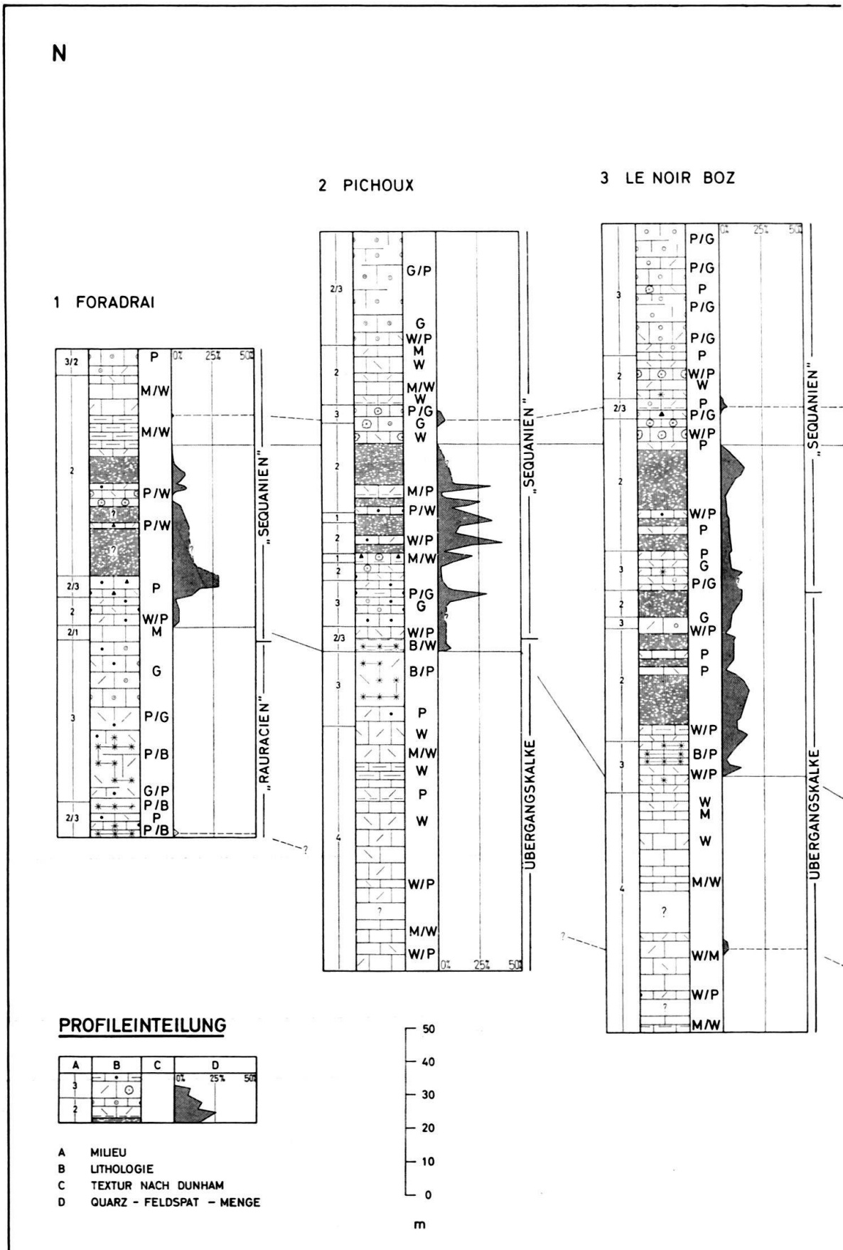
Fig. 2. Westliche Profilerie mit chronostratigraphischen Korrelationen. Erklärung von Milieu- und Textursymbolen siehe Fig. 3.
