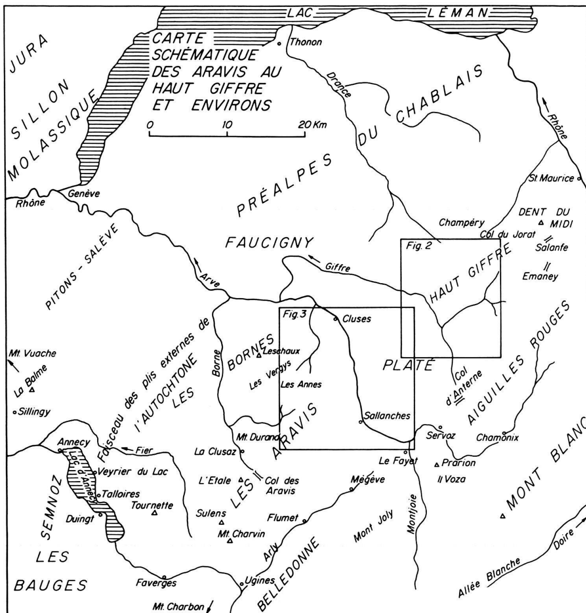
Fig.1 Carte schématique des Aravis au Haut Giffre et environs
