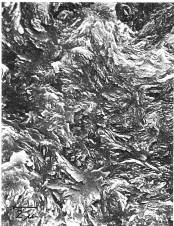
Fig. 19. Gebrochenes Glaukonitkorn. Stereoscan-EM, Probe P/16.
