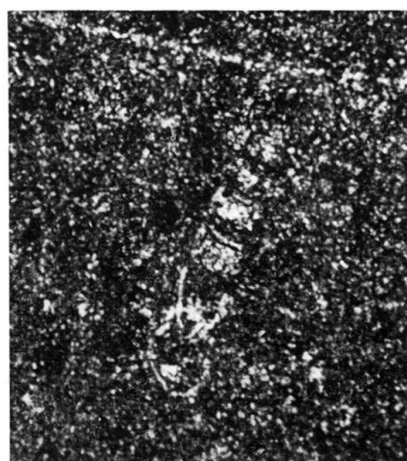
Fig. 2. Microfossile découvert dans le niveau calcaire partiellement dolomitique, au toit du Trias autochtone, couverture du massif des Aiguilles-Rouges. Col de Salenton, Hte-Savoie, France. Coupe mince n. 14. Longueur: env. 0,080 mm.
